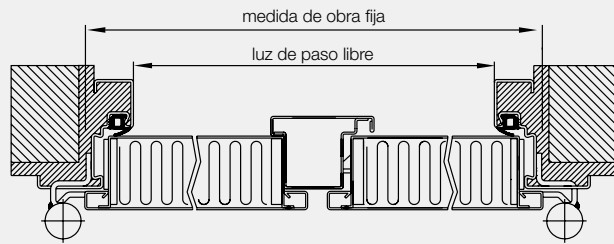
Sección horizontal
