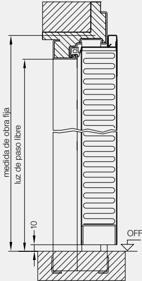
Sección vertical
