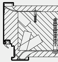
Mampostería anclajes de muro con tacos
