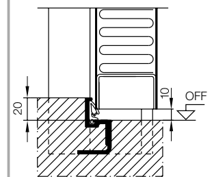
carril de tope con junta
