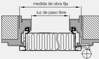
Sección horizontal
