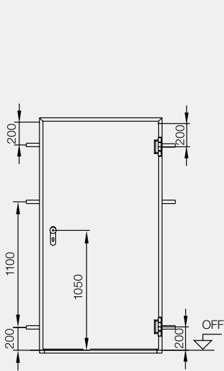
Perspectiva de puerta de 1 hoja
