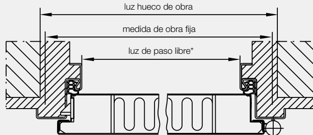
Sección horizontal
