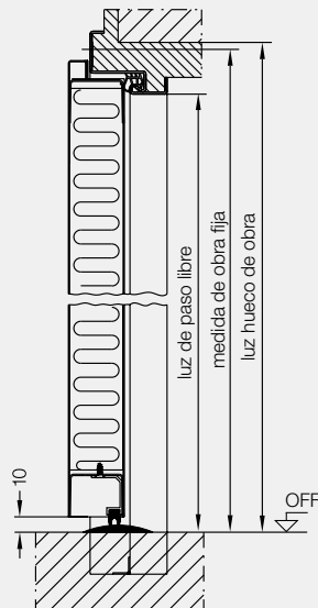
Sección vertical
