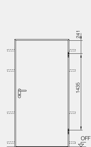
Perspectiva de puerta de 1 hoja
