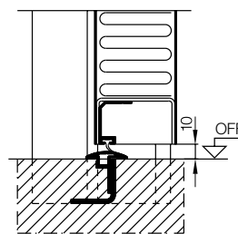
perfil de remate de aluminio con junta, cerco con umbral de retención
