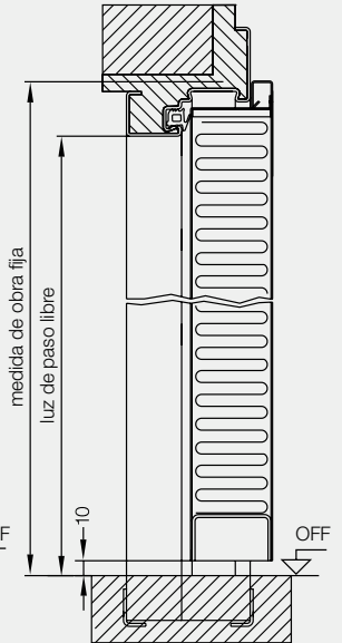
Sección vertical
