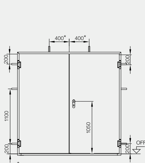
Perspectiva de puerta de 2 hojas
